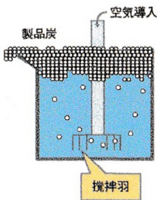
図 4. 浮遊選鉱法
